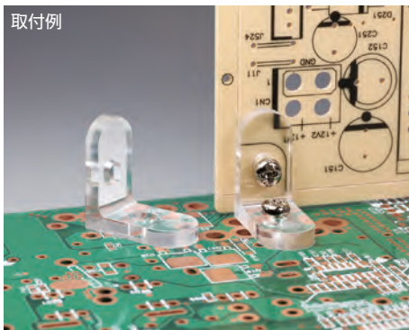
取付例
